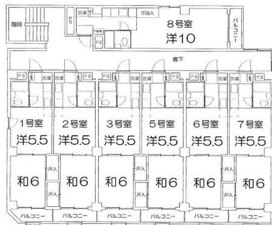
【2階・3階 平面図】
